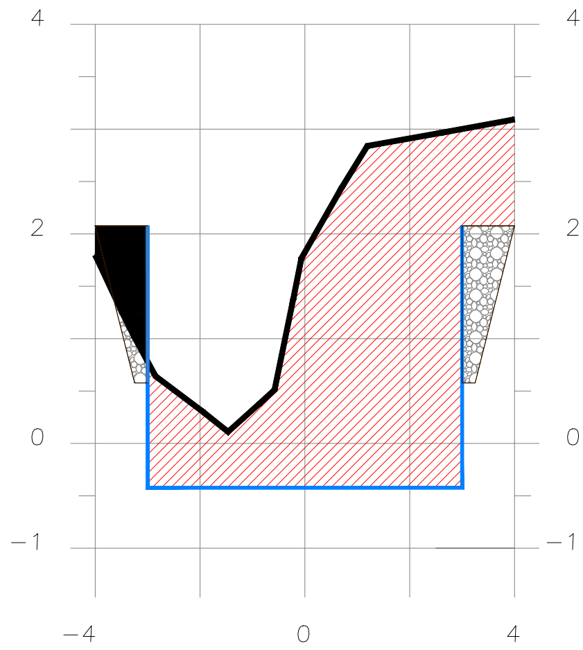
SECCION 2+745
