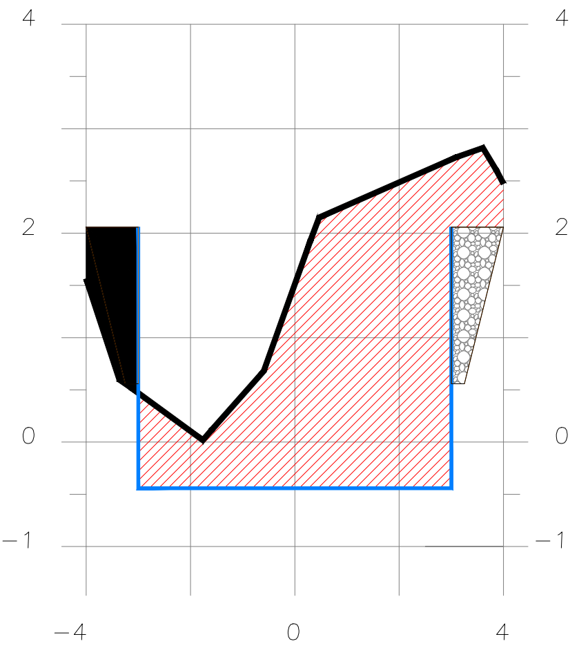
SECCION 2+790
