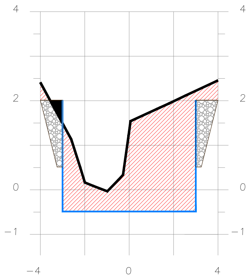
SECCION 2+895
