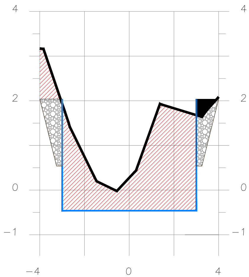
SECCION 2+835
