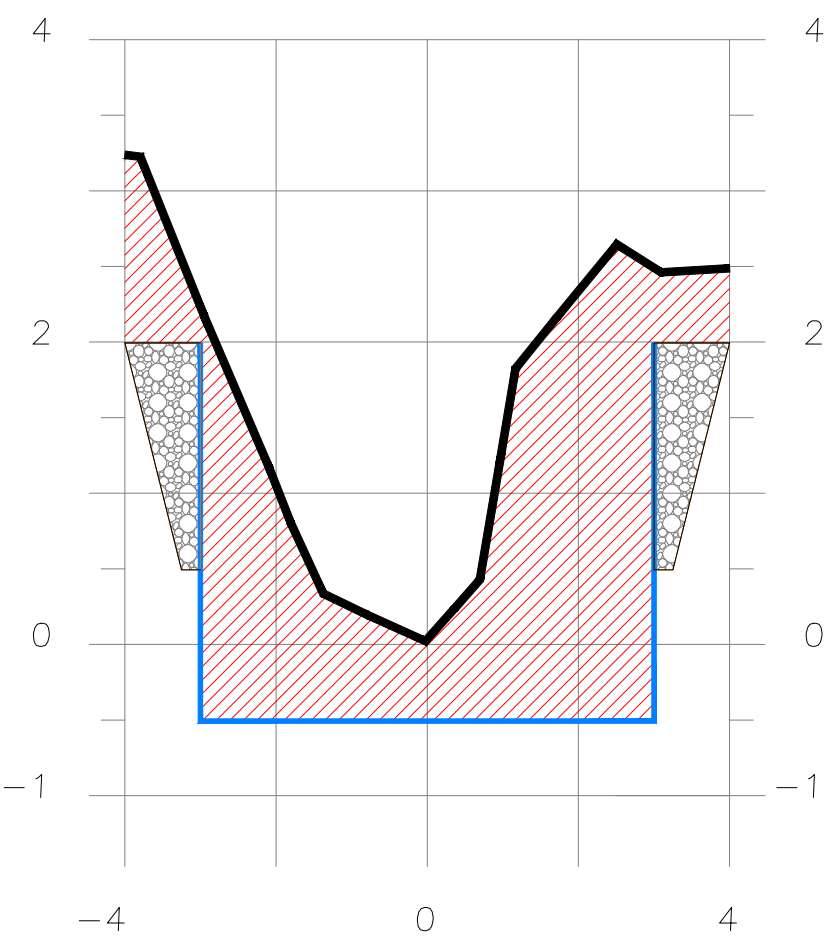
SECCION 2+940
