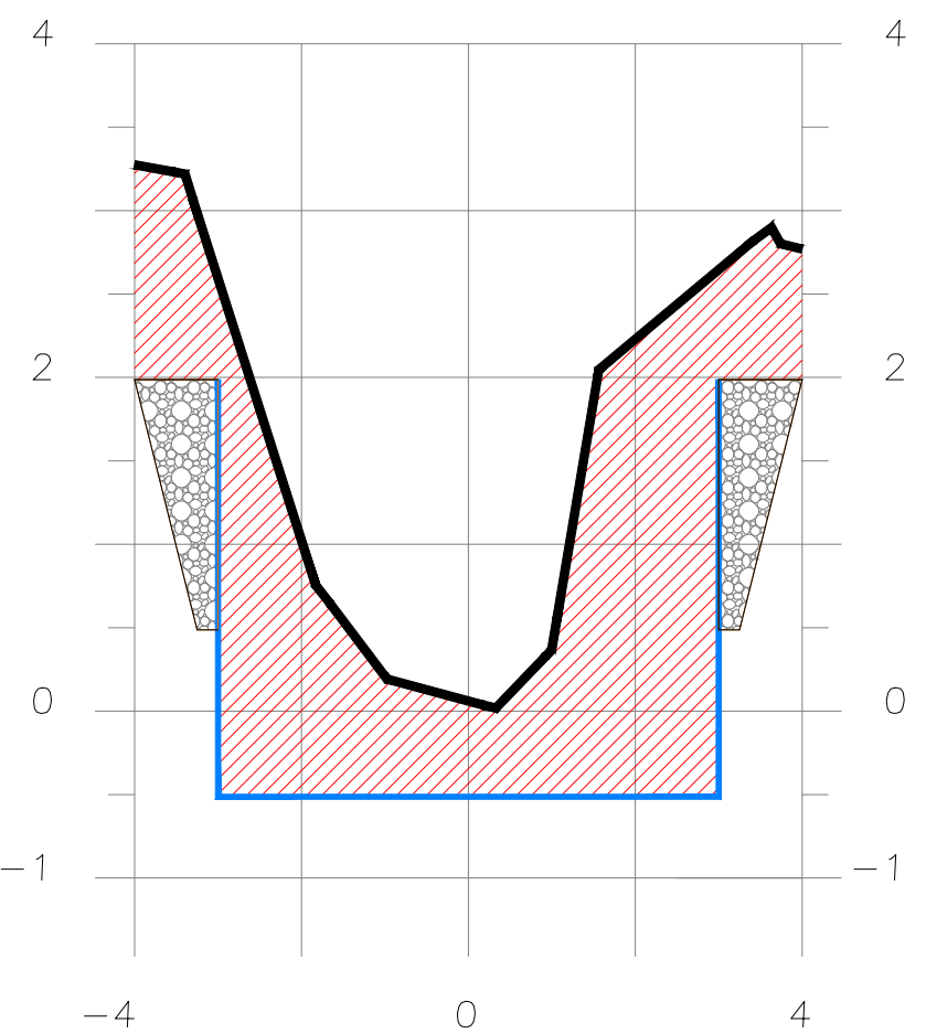
SECCION 2+995
