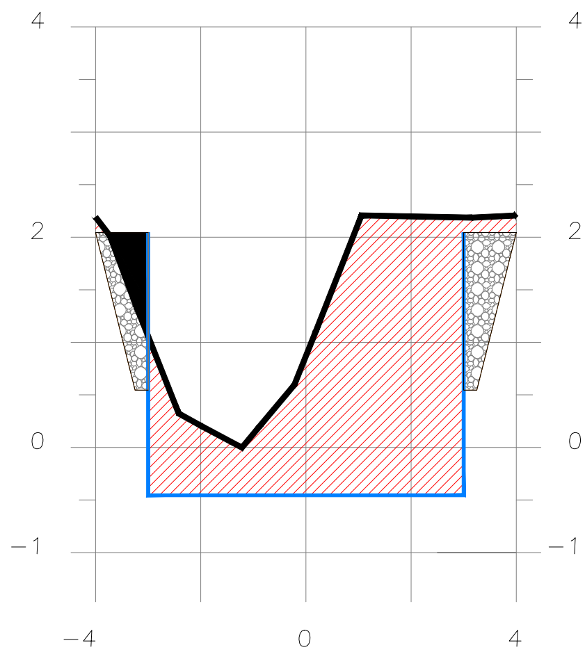
SECCION 2+820
