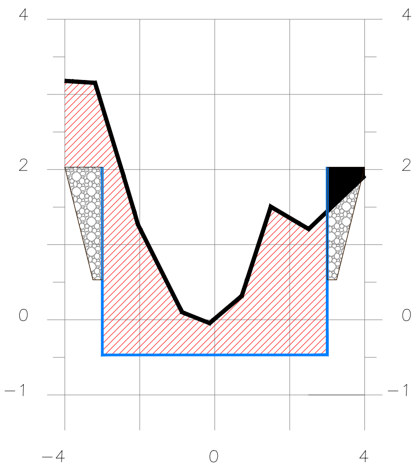
SECCION 2+850
