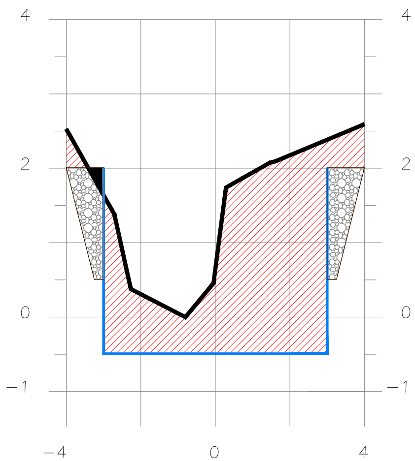
SECCION 2+910
