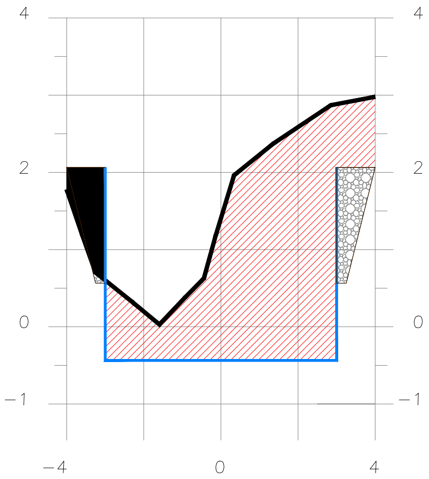
SECCION 2+775
