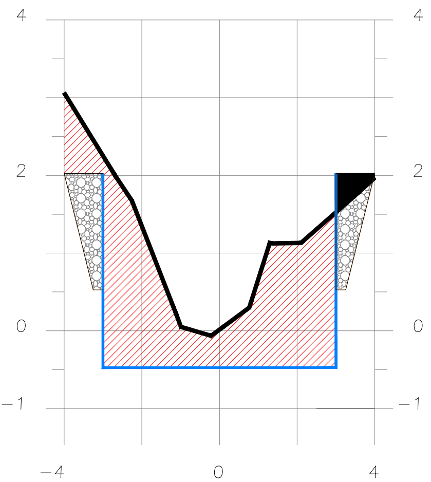
SECCION 2+865
