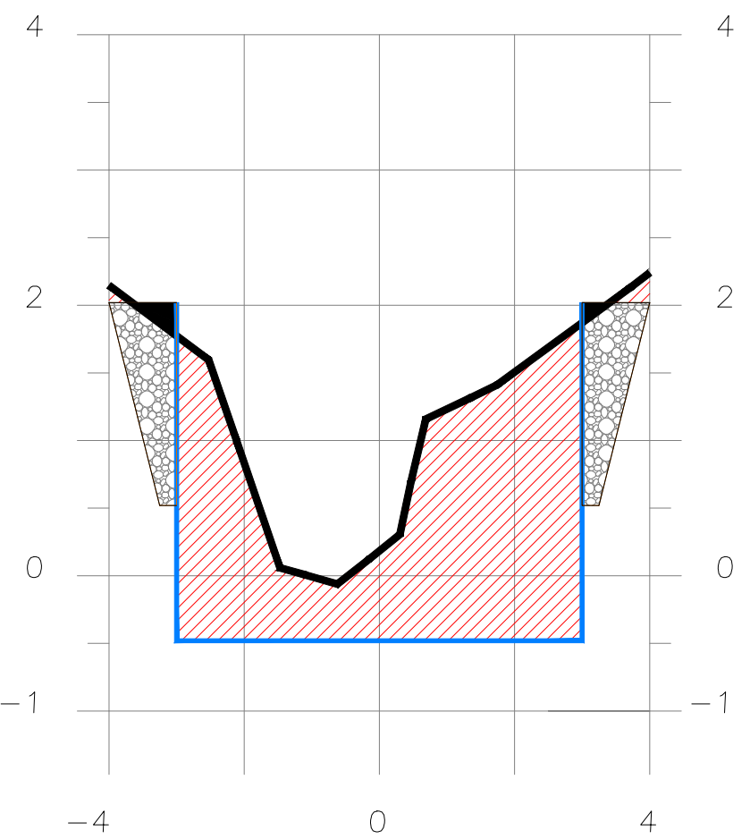
SECCION 2+880
