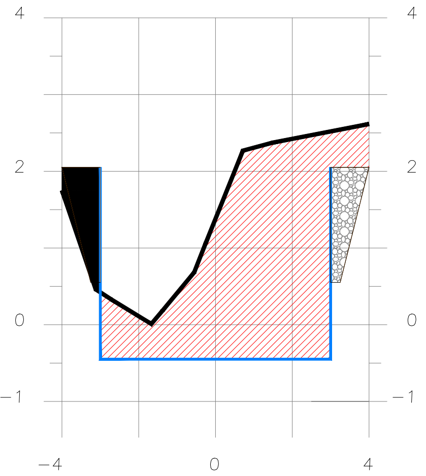
SECCION 2+805
