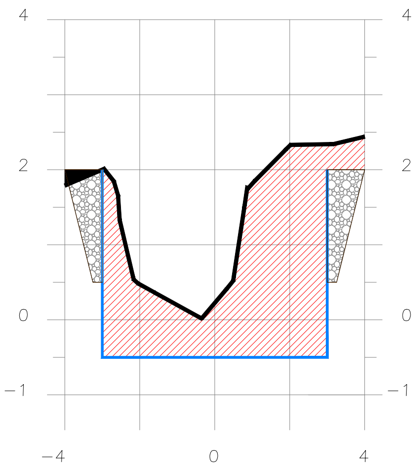
SECCION 2+925
