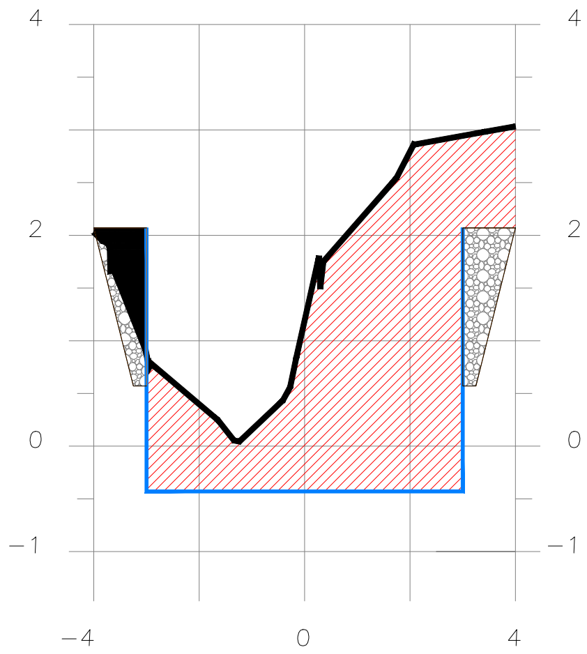
SECCION 2+760
